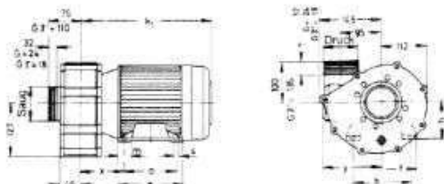
Dimensiones BADU 21-80/31 • 21-80/34 G
