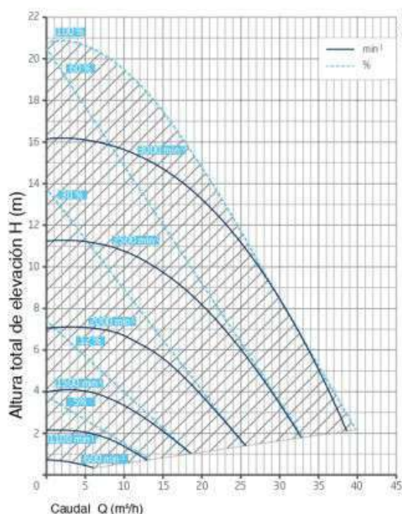
Curvas de rendimiento
