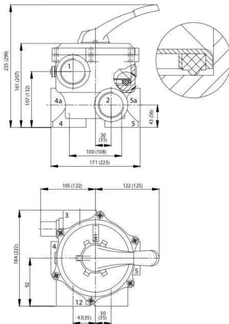
Esquema de dimensiones (en mm)
